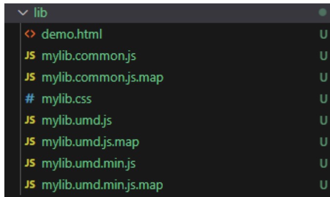
图 1-10 输出件
