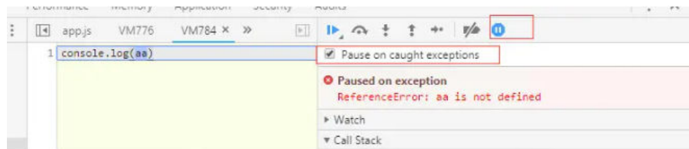
图 1-24 异常断点
