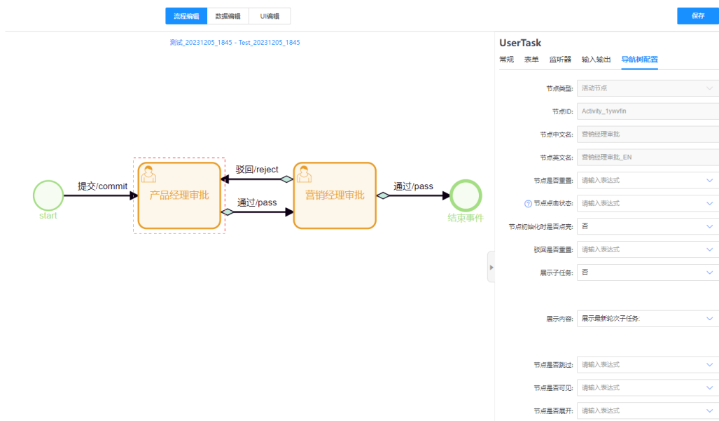
图 3-52 导航树配置
