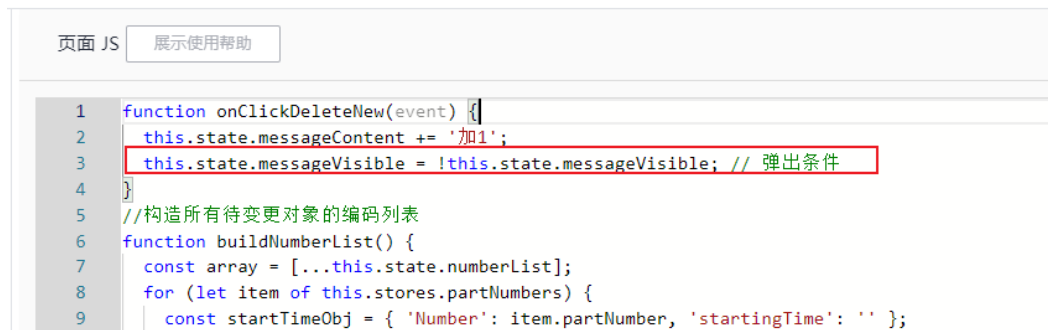
图 3-120 按条件提示
