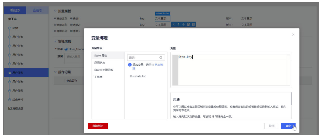
图 3-141 循环渲染
