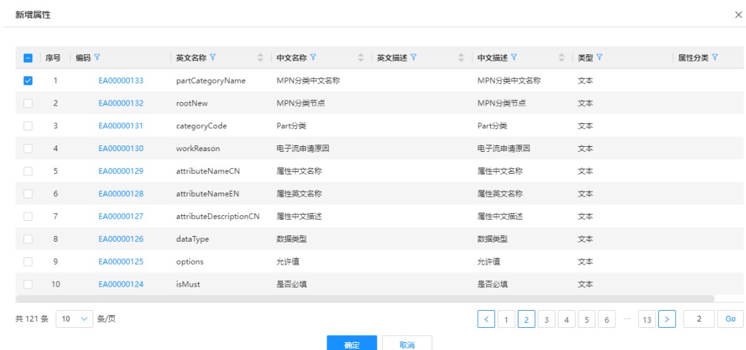
图 3-64 新增属性
