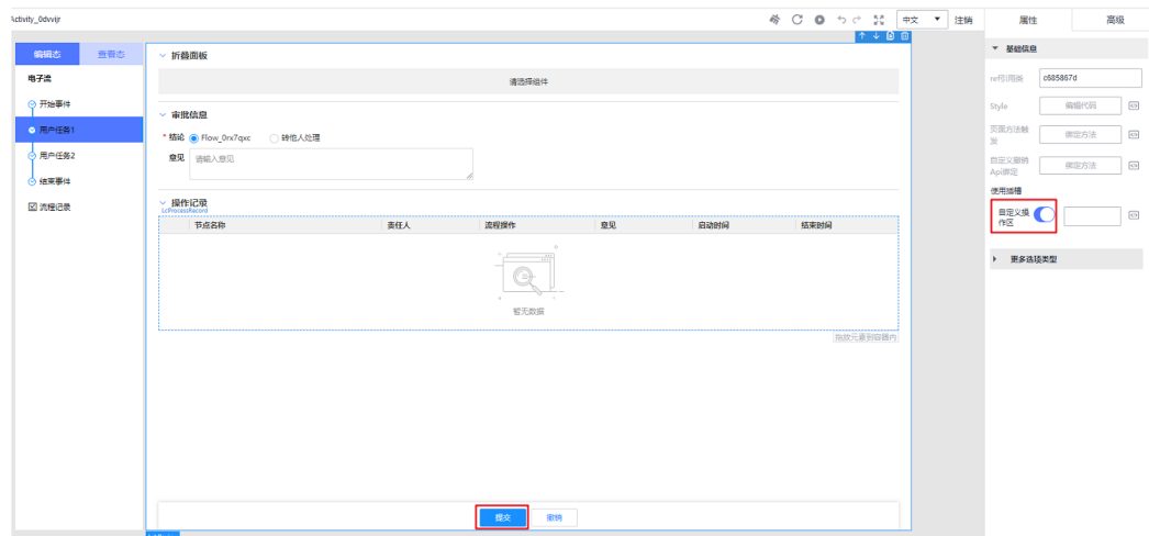
图 3-37 提交按钮
