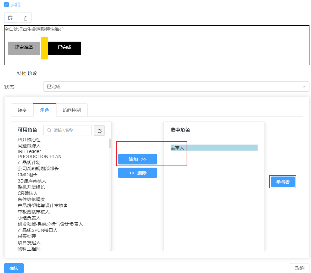
图 4-8
