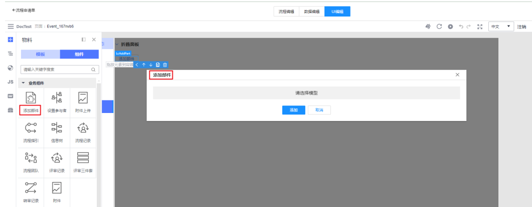
图 3-27 添加部件
