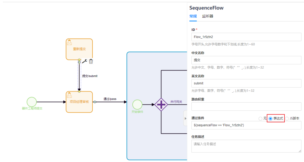
图 3-3 通过条件
