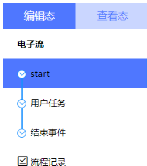
图 3-83 导航树
