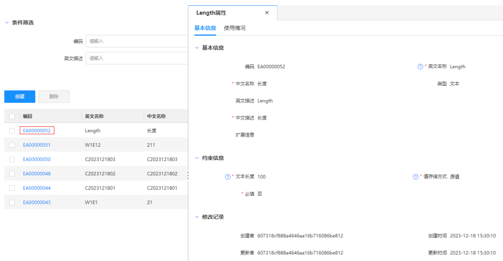
图 3-61 基本信息
