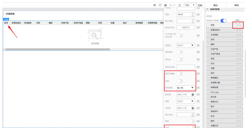
图 3-25 设置表字段
