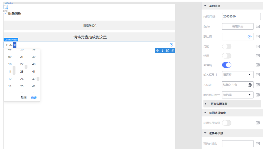
图 3-124 时间选择器
