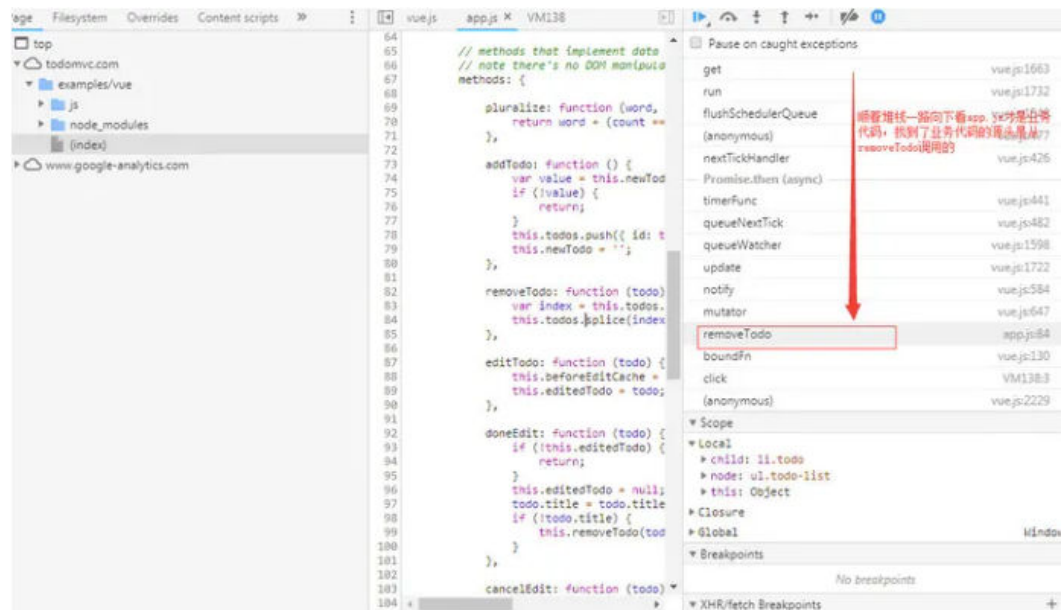
图 1-21 代码追溯
