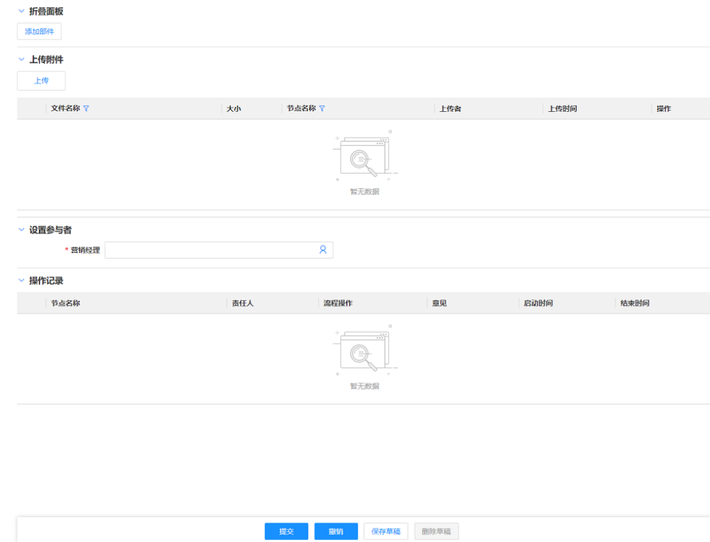
图 3-84 画布
