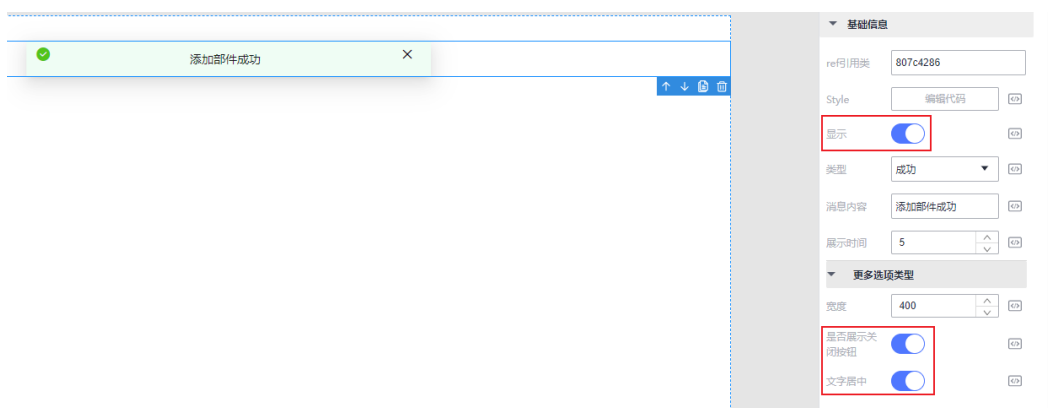
图 3-119 消息提示框
