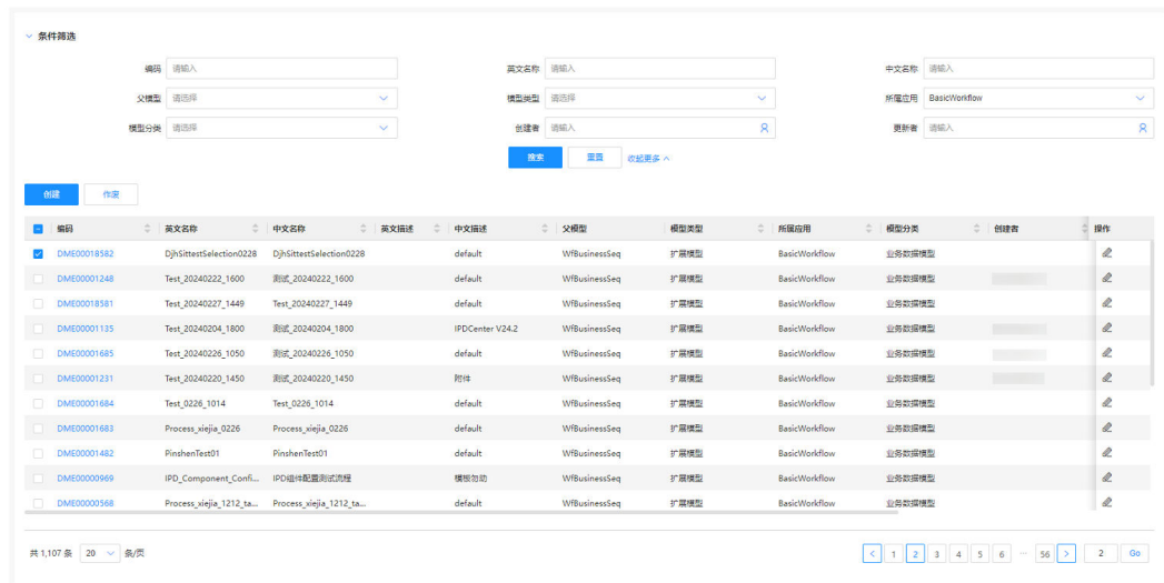
图 3-66 条件筛选
