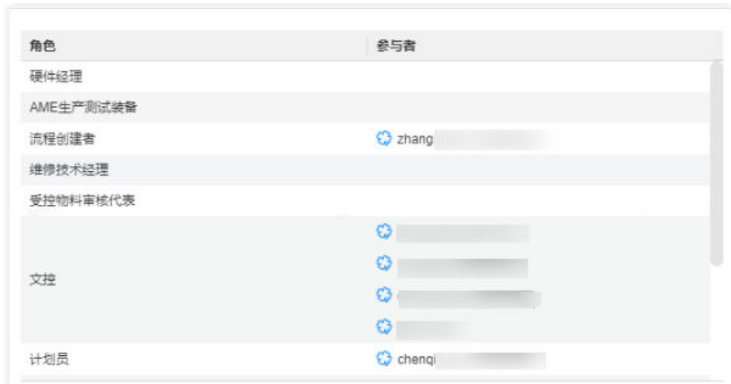
图 3-91 团队角色
