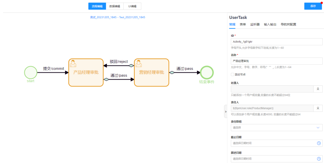
图 3-50 属性设置
