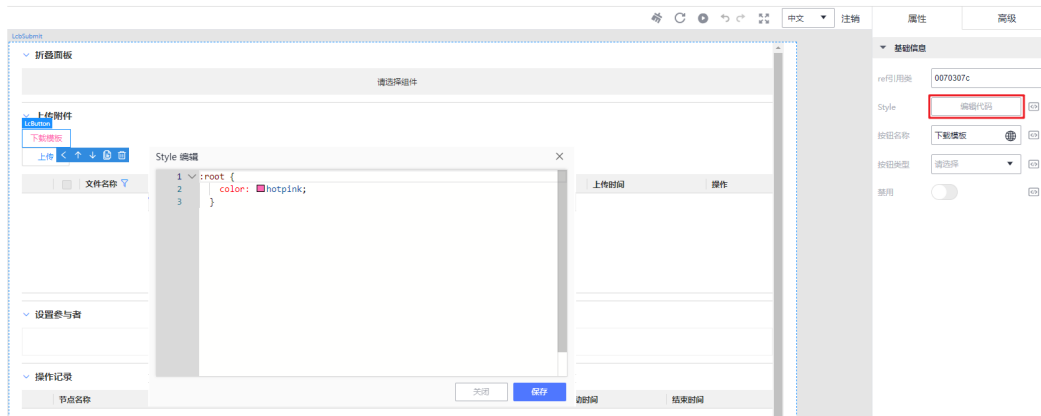
图 3-131 编辑代码
