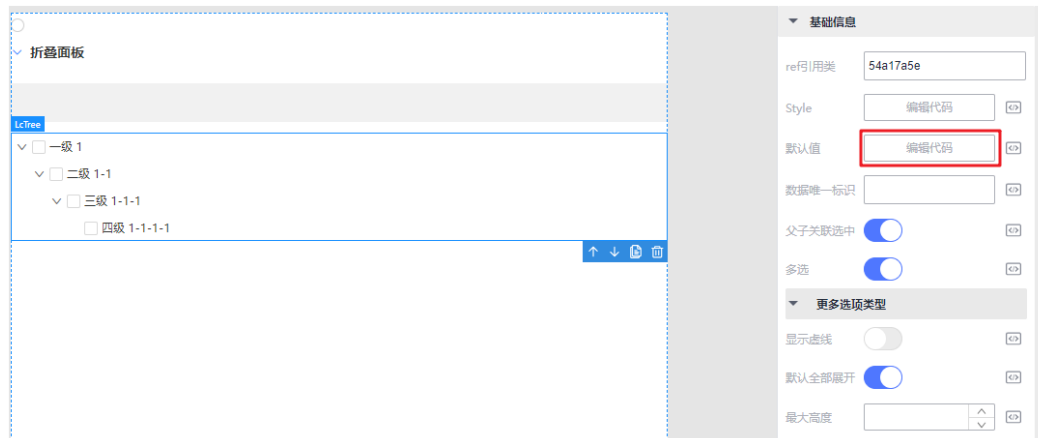
图 3-127 树形展示
