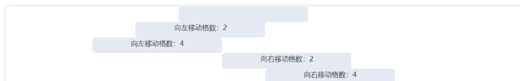
图 3-100 移动格数
