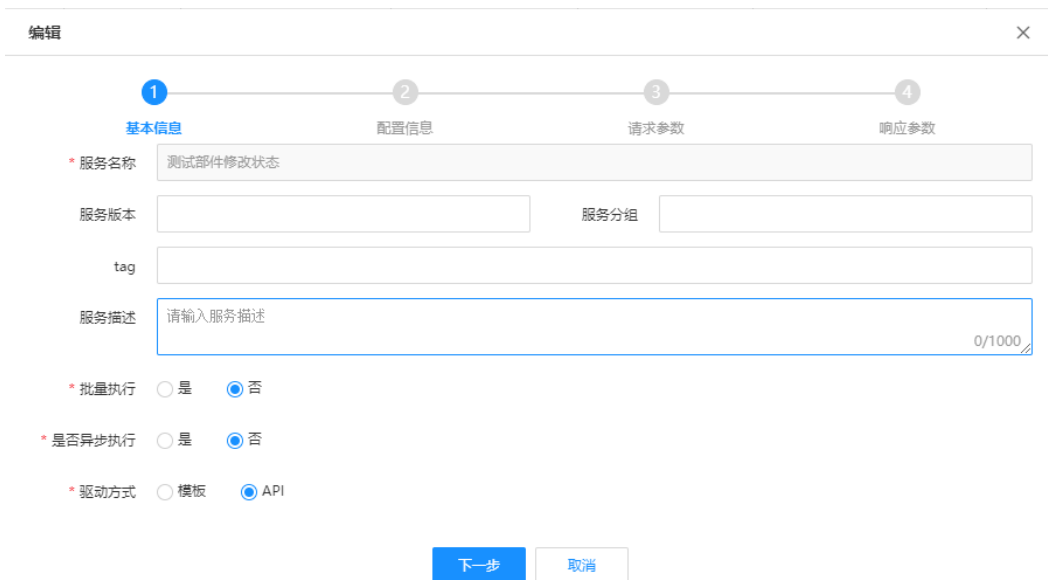
图 3-6 基本信息
