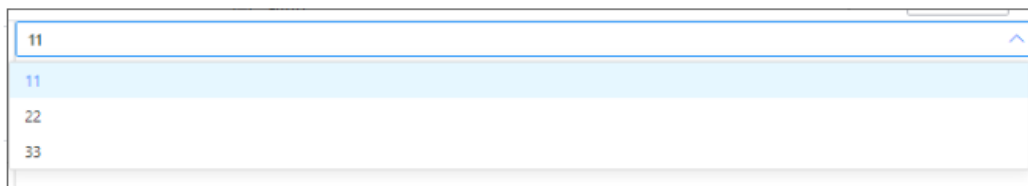
图 3-123 选项展示
