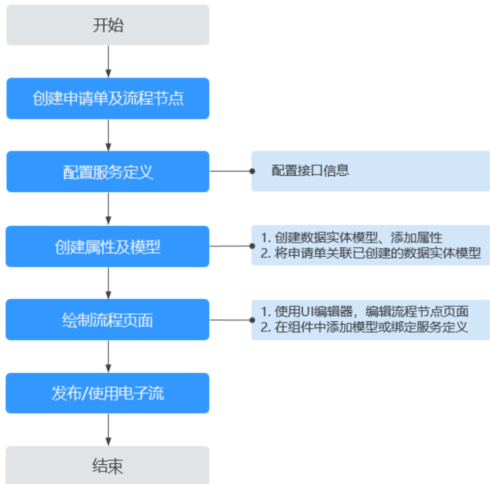
图 3-1 操作流程
