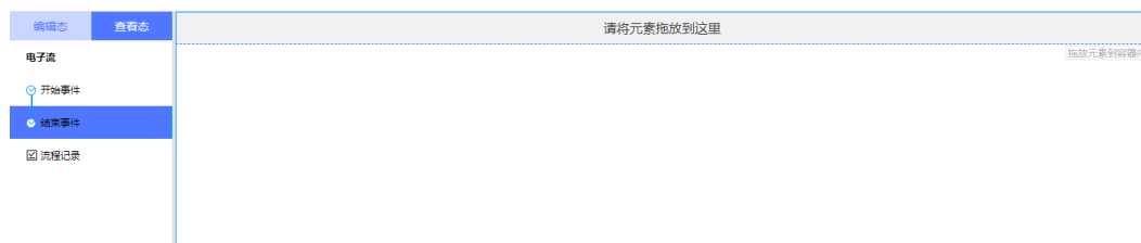
图 3-97 BOX 组件
