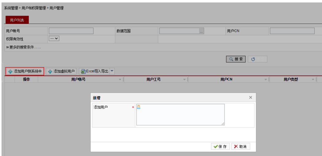
图 4-17 添加用户
