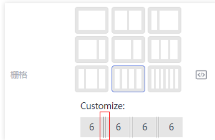
图 3-102 栅格
