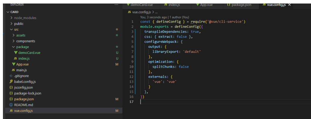
图 1-8 vue.config.js 配置
