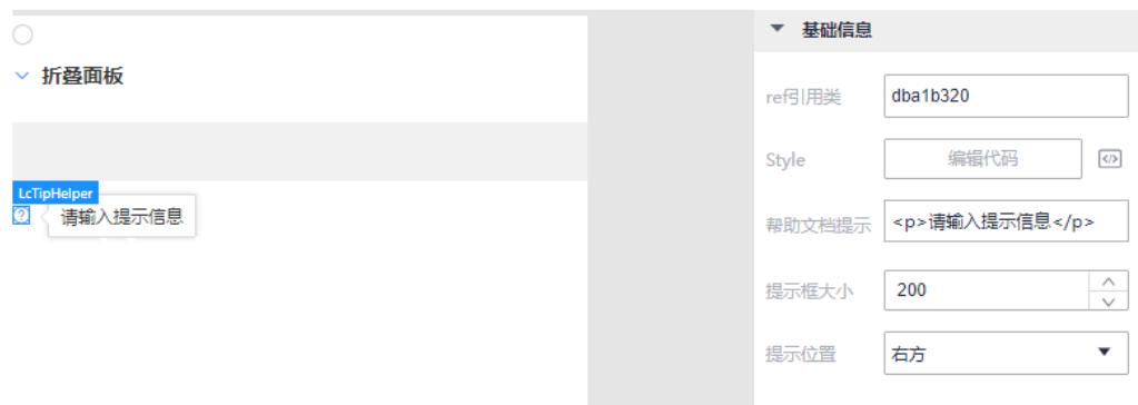
图 3-117 提示位置
