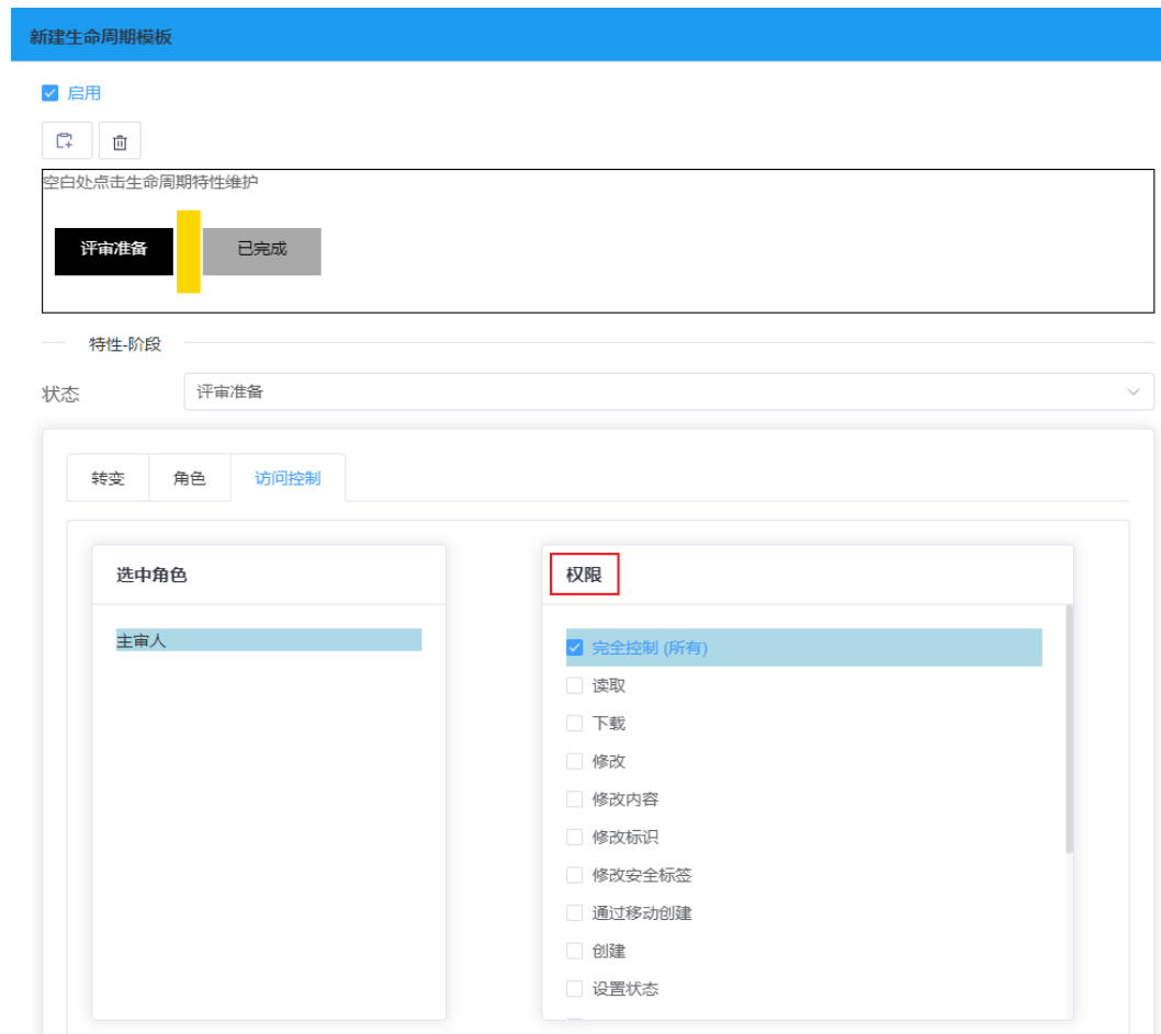
图 4-9 添加权限
