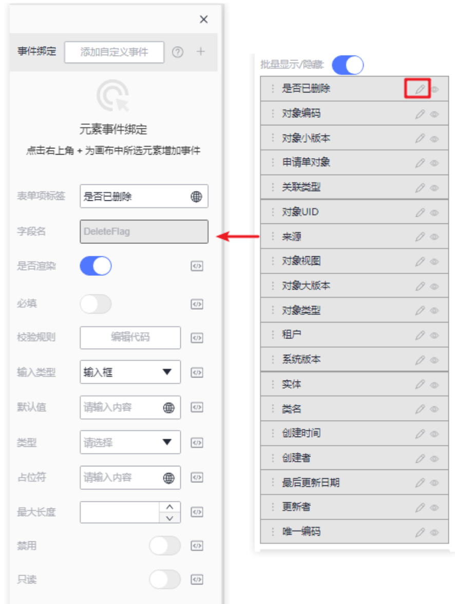
图 3-126 表单项
