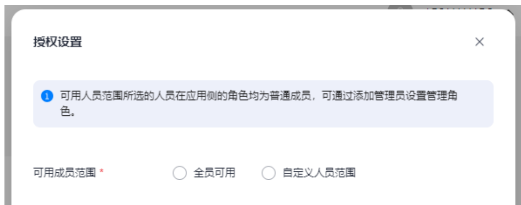
图 2-4 授权设置-2
