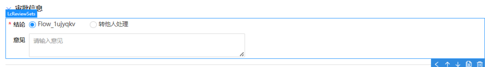
图 3-89 移动组件
