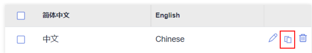
图 3-149 复制键值
