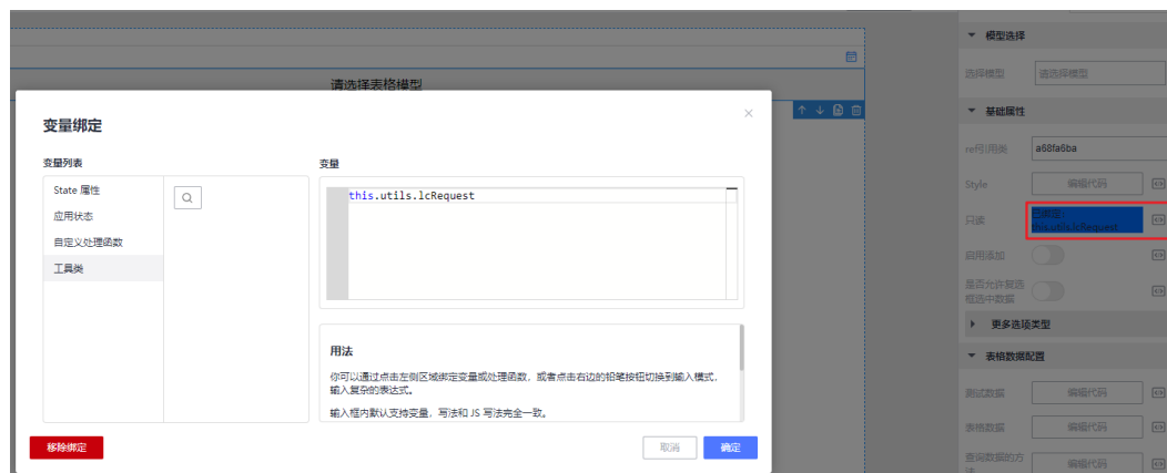
图 3-139 绑定变量
