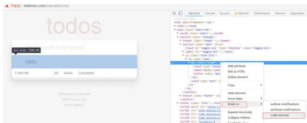
图 1-22 Dom 断点
